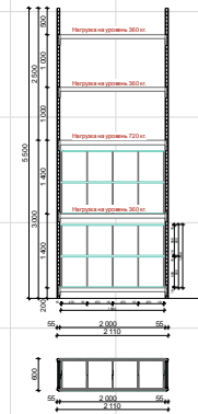
Тип №2 грузовой стеллажа.
