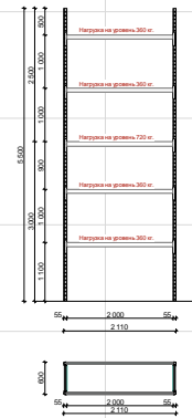
Тип №1 грузовой стеллажа.
